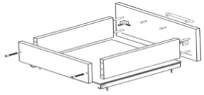
Сборка ящиков
