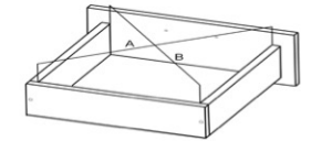
Сборка ящиков
