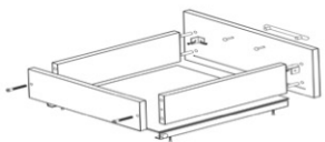
Сборка ящиков
