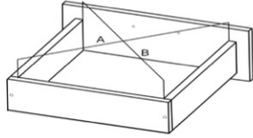
Сборка ящиков
