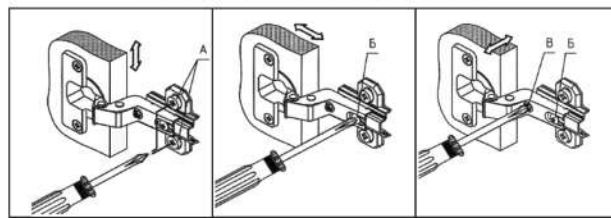
Регулювання завісів - Регулировка петель
