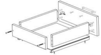
Сборка ящиков
